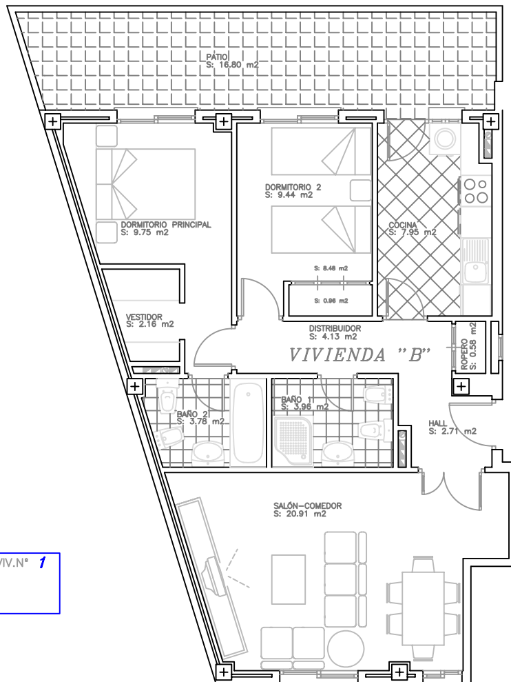
PLANTA BAJA, PISO "B" - PORTAL 1
