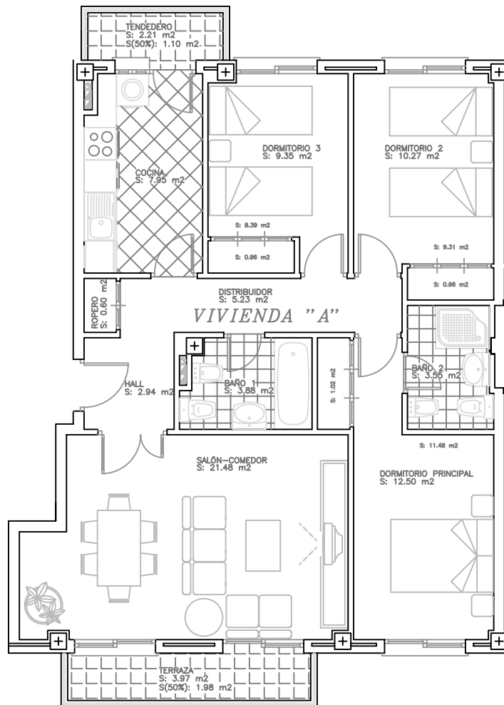
PLANTA SEGUNDA, PISO "A" - PORTAL 1
