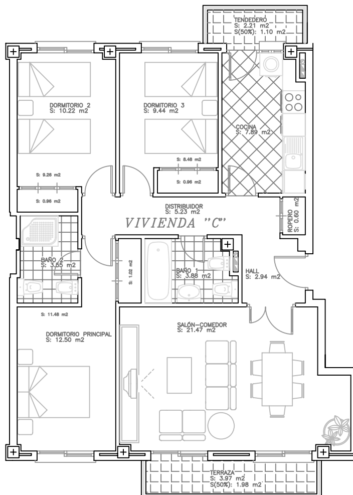
PLANTA SEGUNDA, PISO "C" - PORTAL 2
