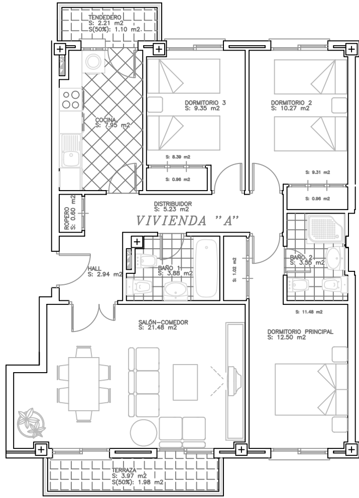
PLANTA PRIMERA, PISO "A" - PORTAL 1
